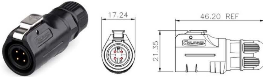
LP-12-C__PE-XX-001 Plug
